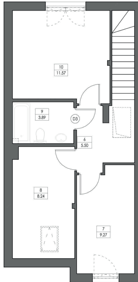
RZUT PIĘTRA
