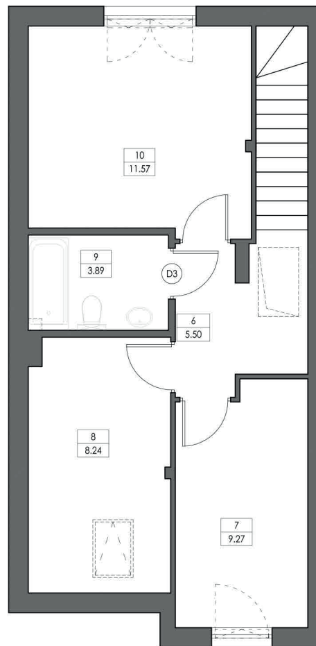
RZUT PIĘTRA
