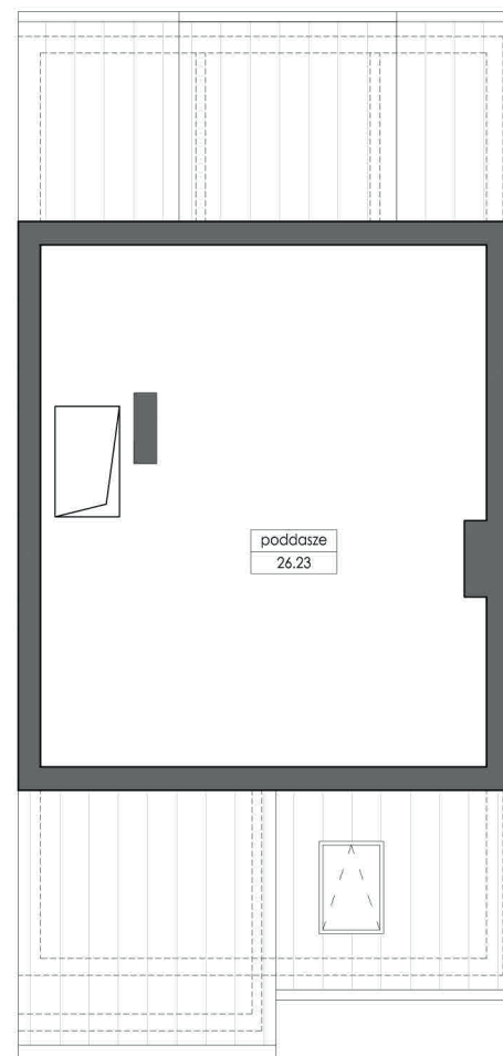
PODDASZE
